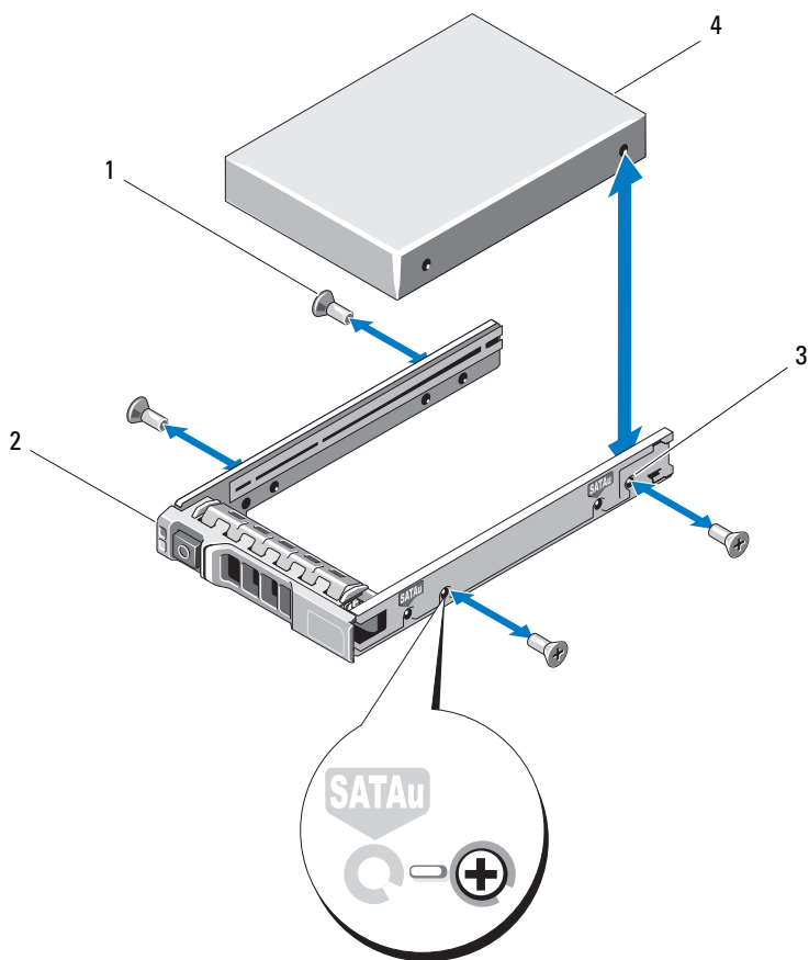
图 16-6. 卸除并安装硬盘驱动器到 2.5 英寸硬盘驱动器托盘中
